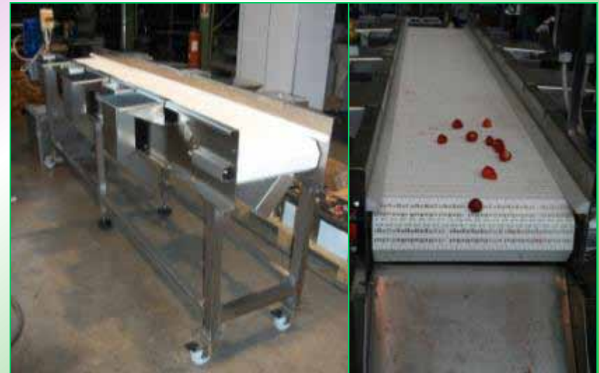
Sortēšanas konveijers
